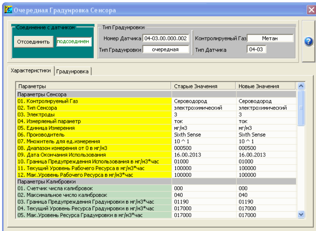
Рисунок Б.9 Страница «Характеристики»
