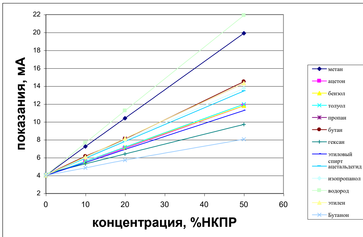
Диаграмма чувствительности измерительного преобразователя ГР1.0 для различных горючих газов и паров, отградуированного по метану.
